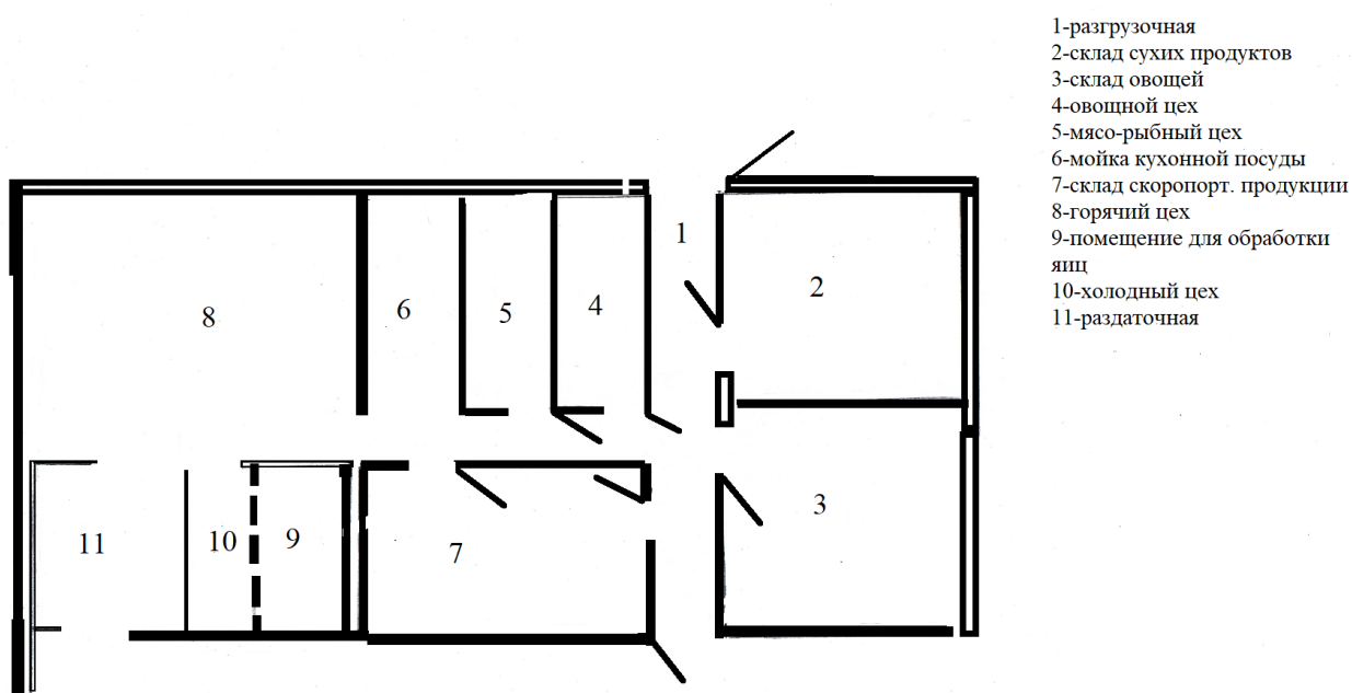
План-схема пищеблока
